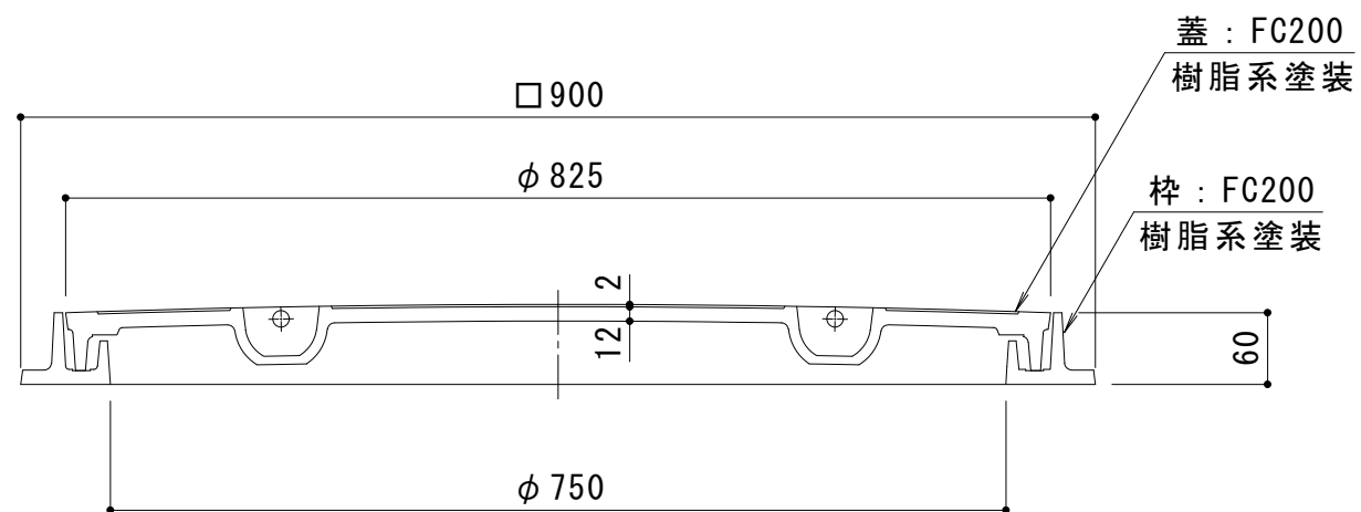
A - A 断面図
