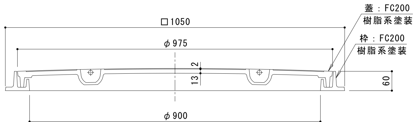
A-A 断面図
