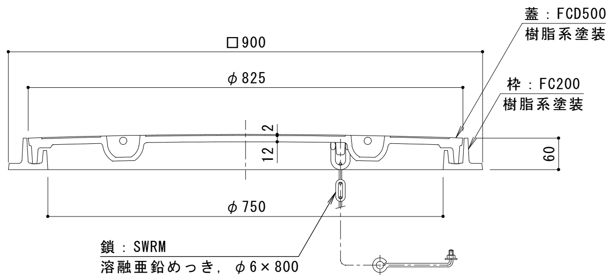
A-A断面図
