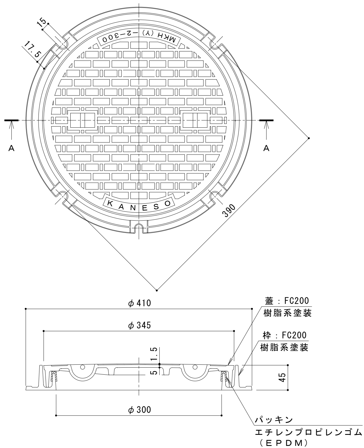
A-A断面図
