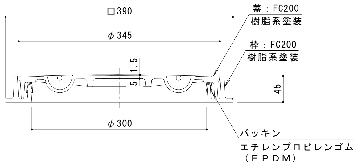
A-A断面図
