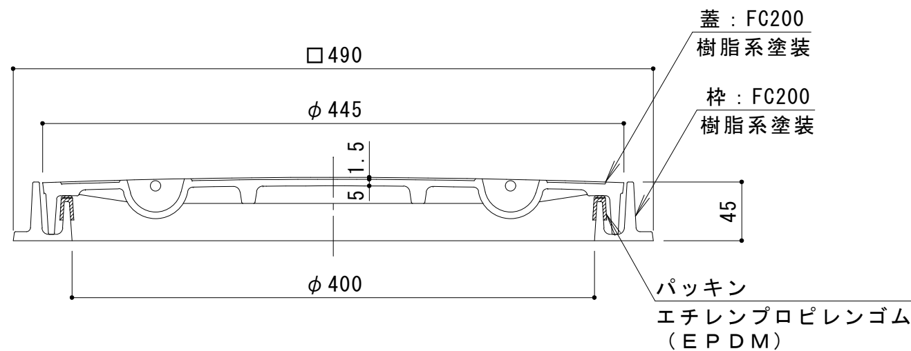
A - A 断面図
