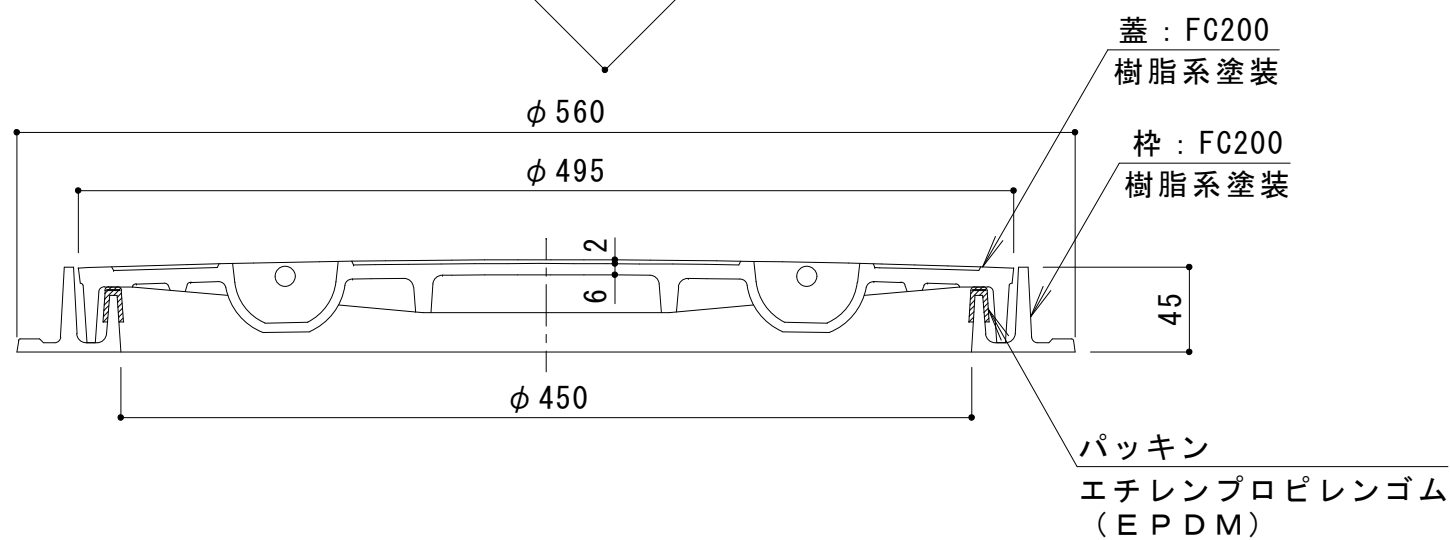
A-A断面図
