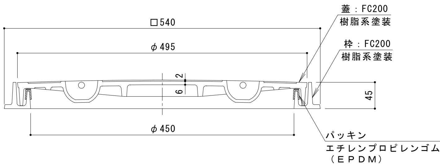
A-A 断面図
