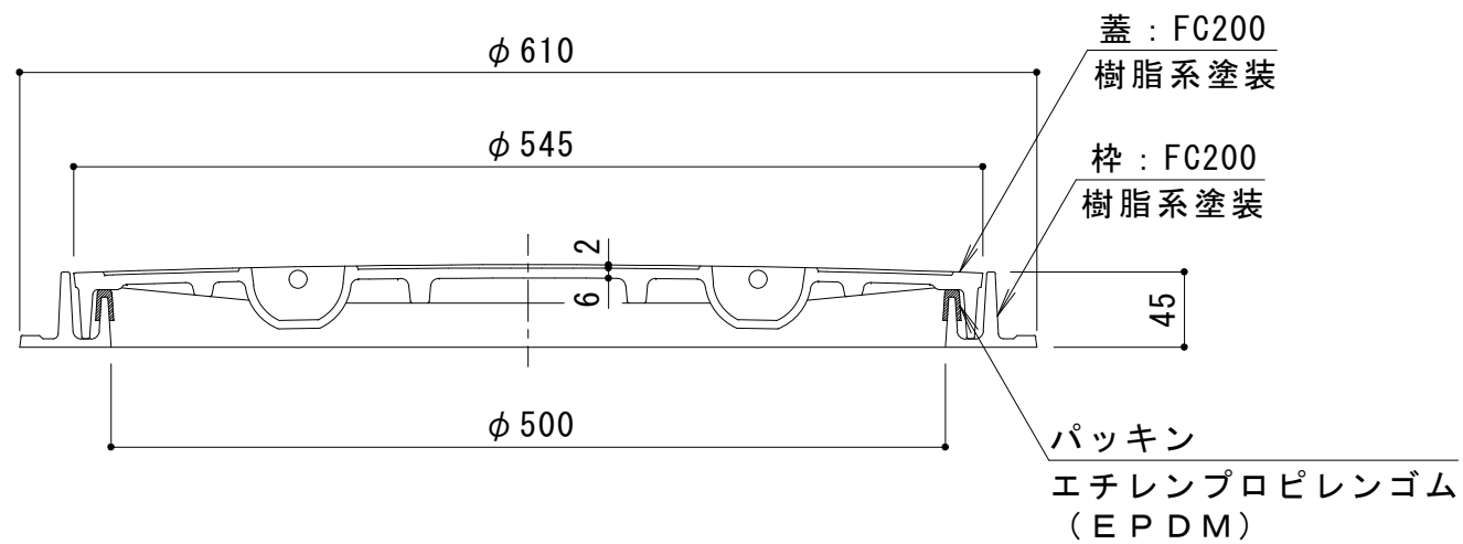
A-A断面図
