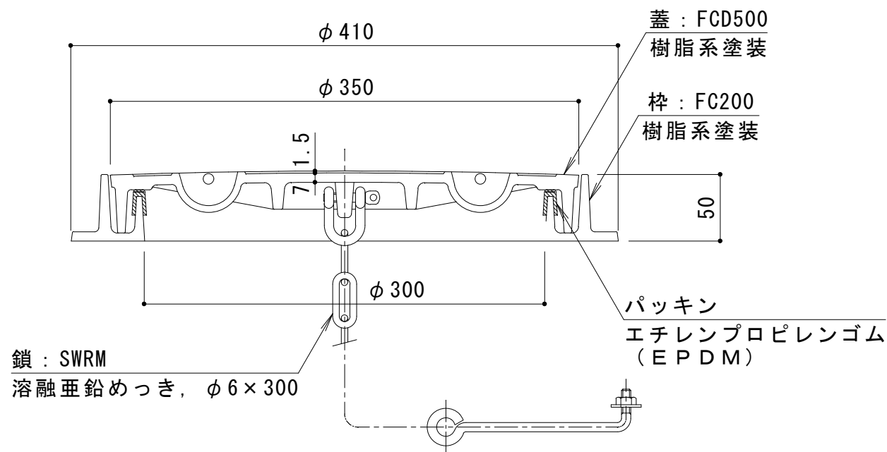
A-A 断面図
