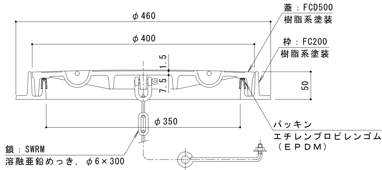
A-A断面図
