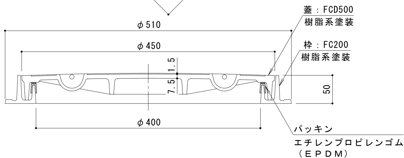
A-A断面図
