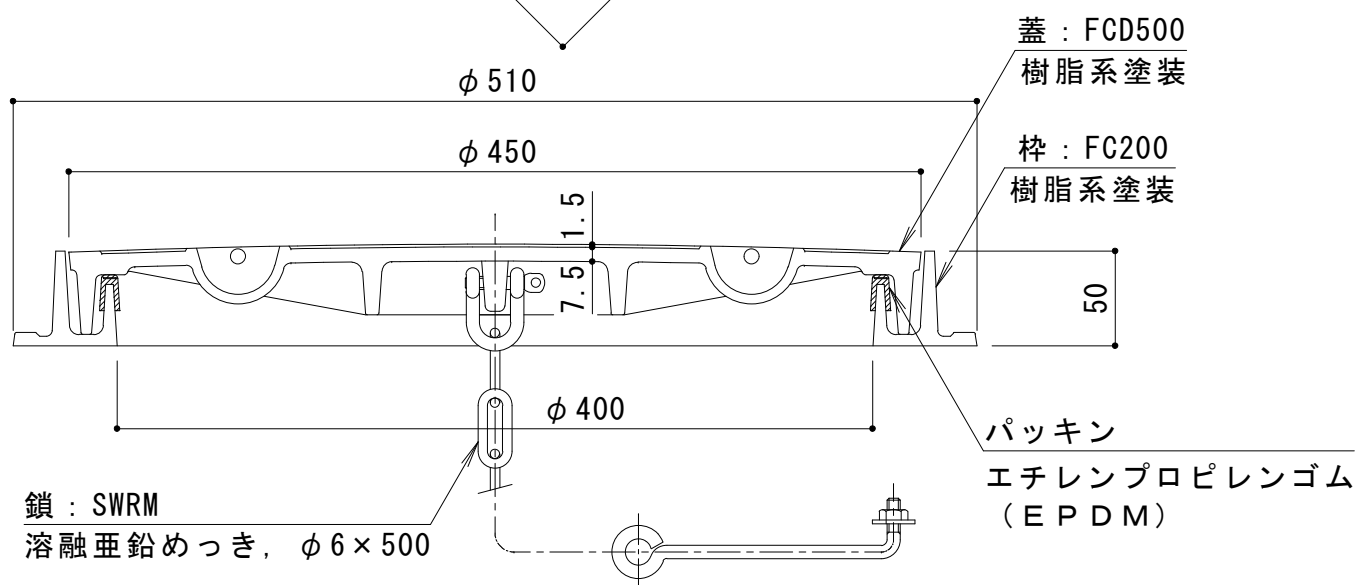
A-A断面図
