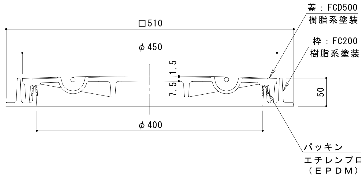
A-A 断面図
