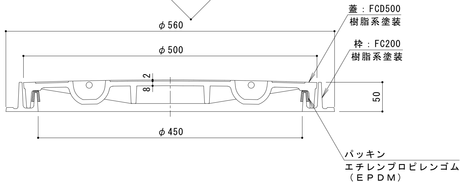
A-A断面図
