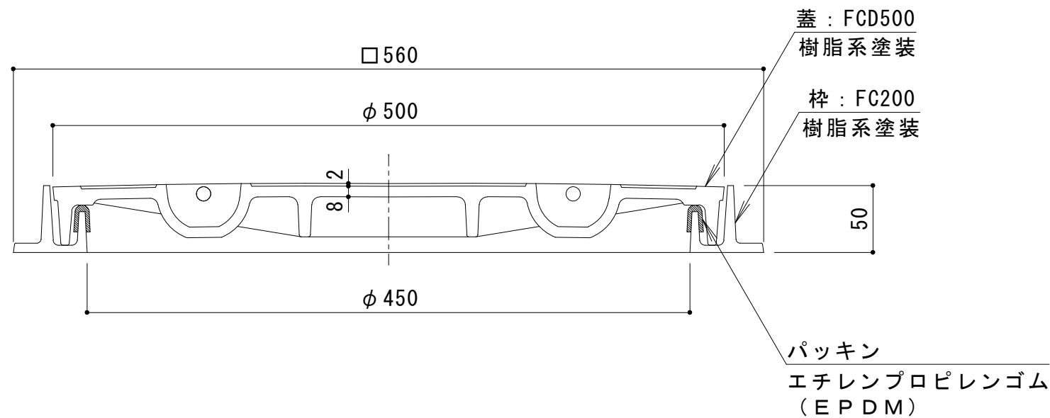
A-A断面図
