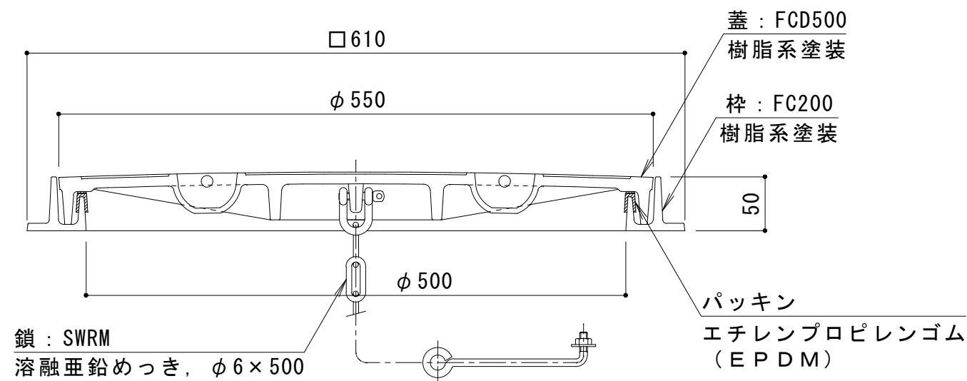
A-A断面図
