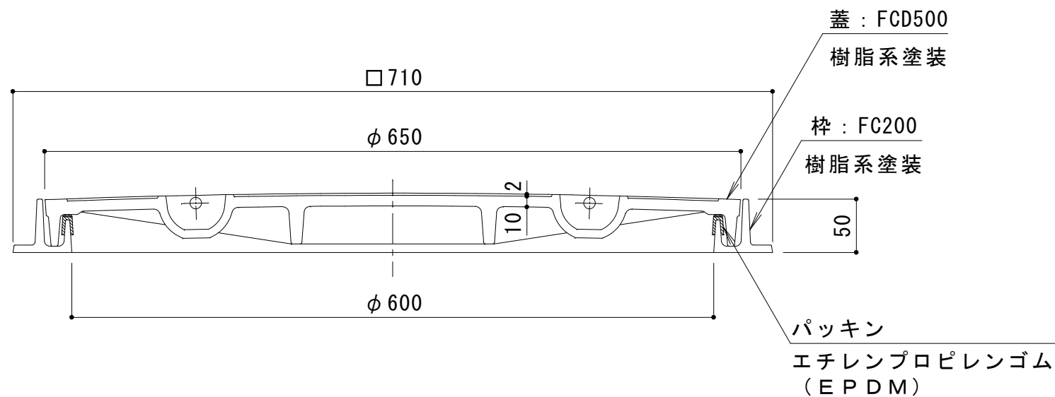
A-A断面図
