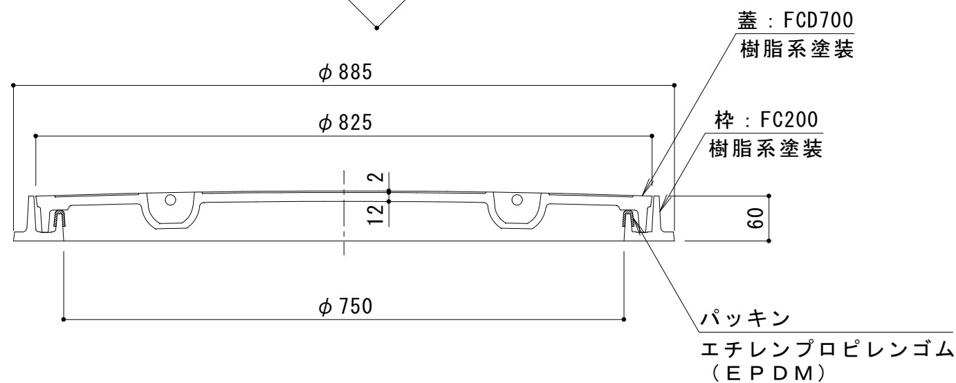
A-A断面図
