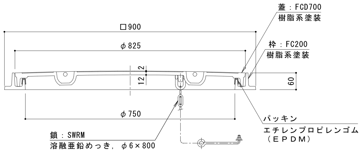
A-A断面図
