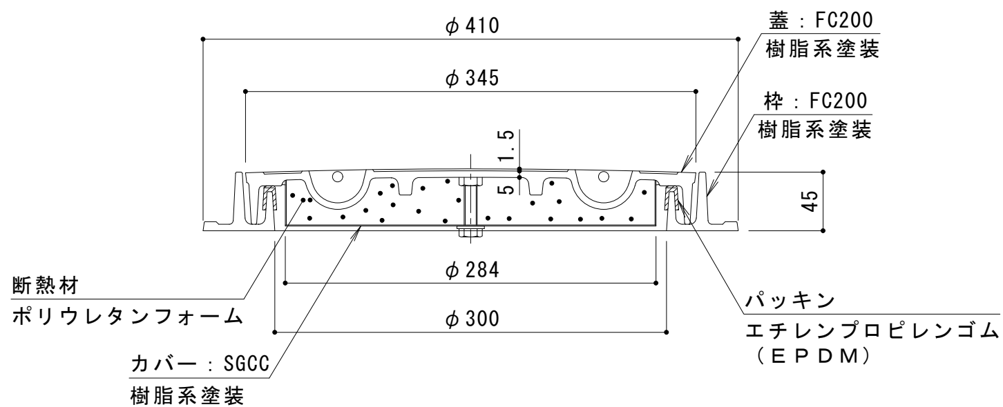
A-A断面図
