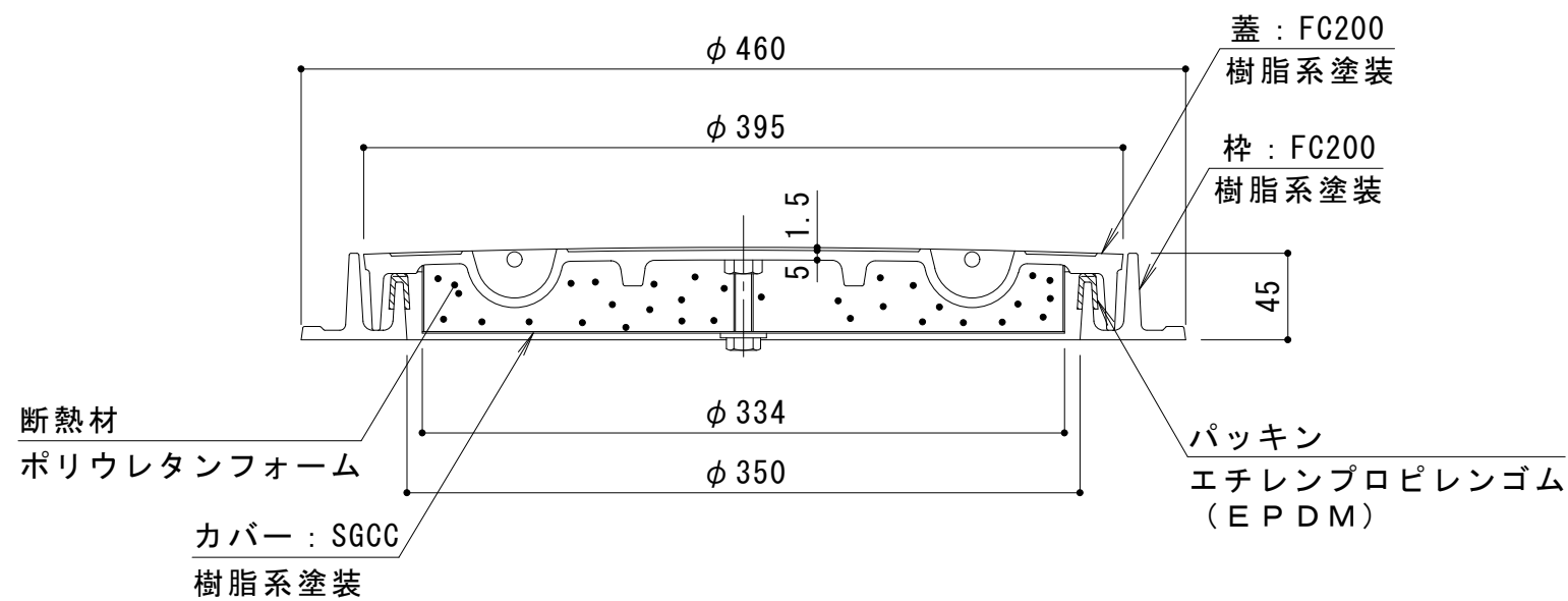
A-A 断面図
