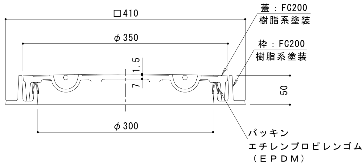
A-A断面図
