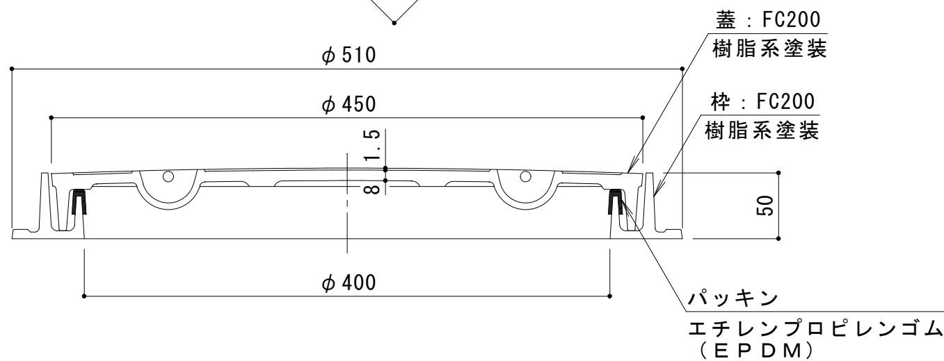
A-A断面図
