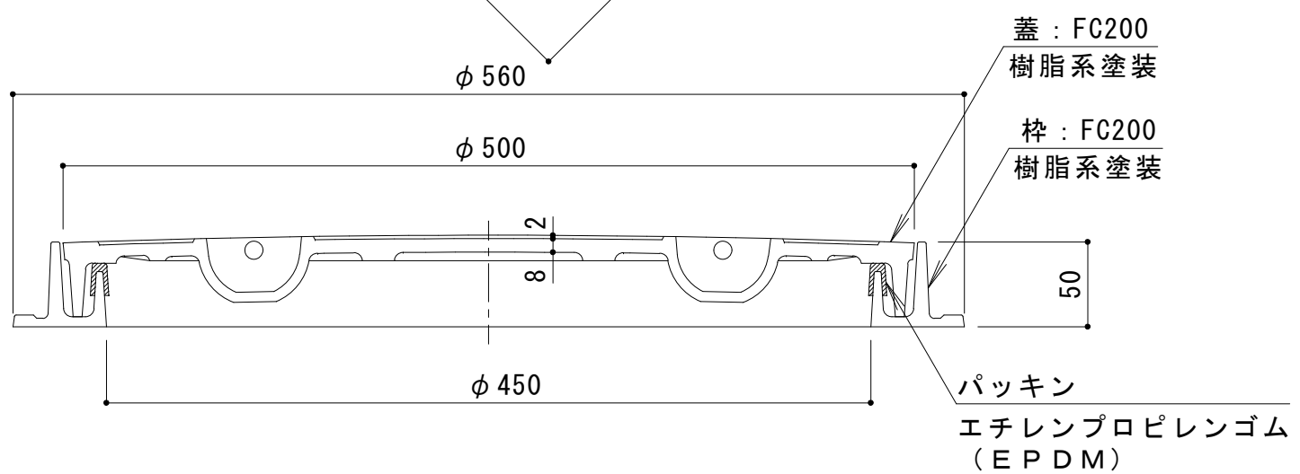
A-A断面図
