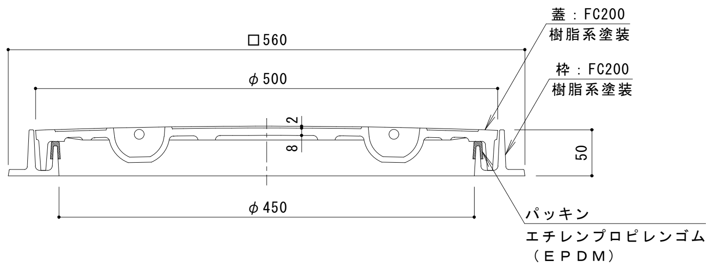
A-A断面図
