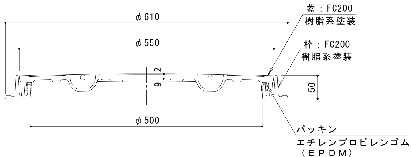
A-A断面図
