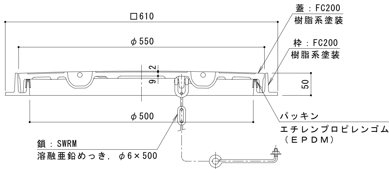
A-A断面図
