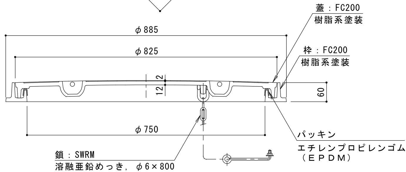
A-A断面図
