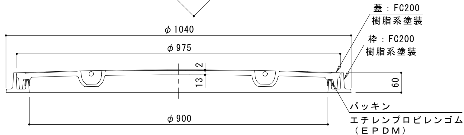
A-A断面図
