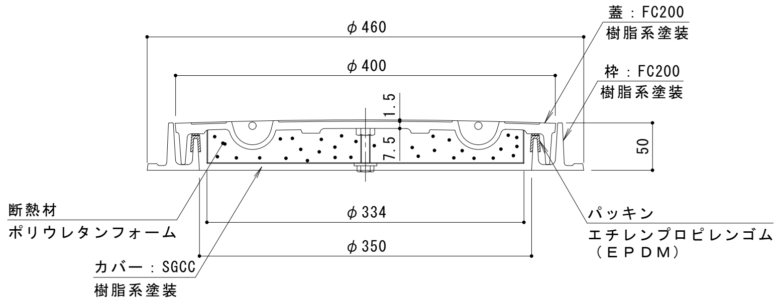
A-A断面図
