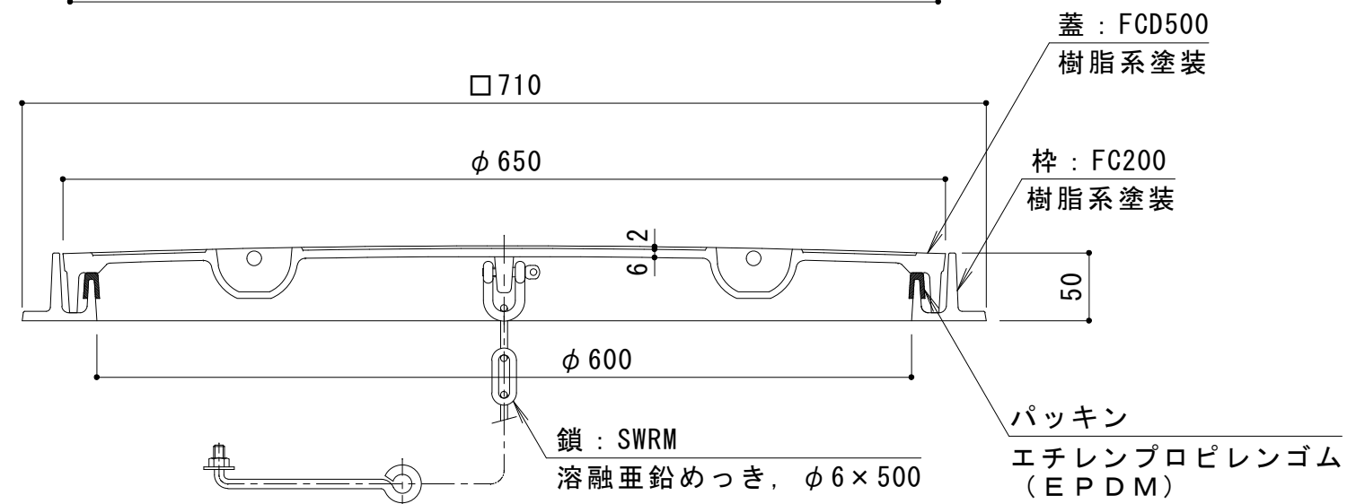
A-A断面図
