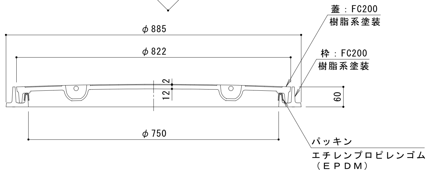
A-A断面図
