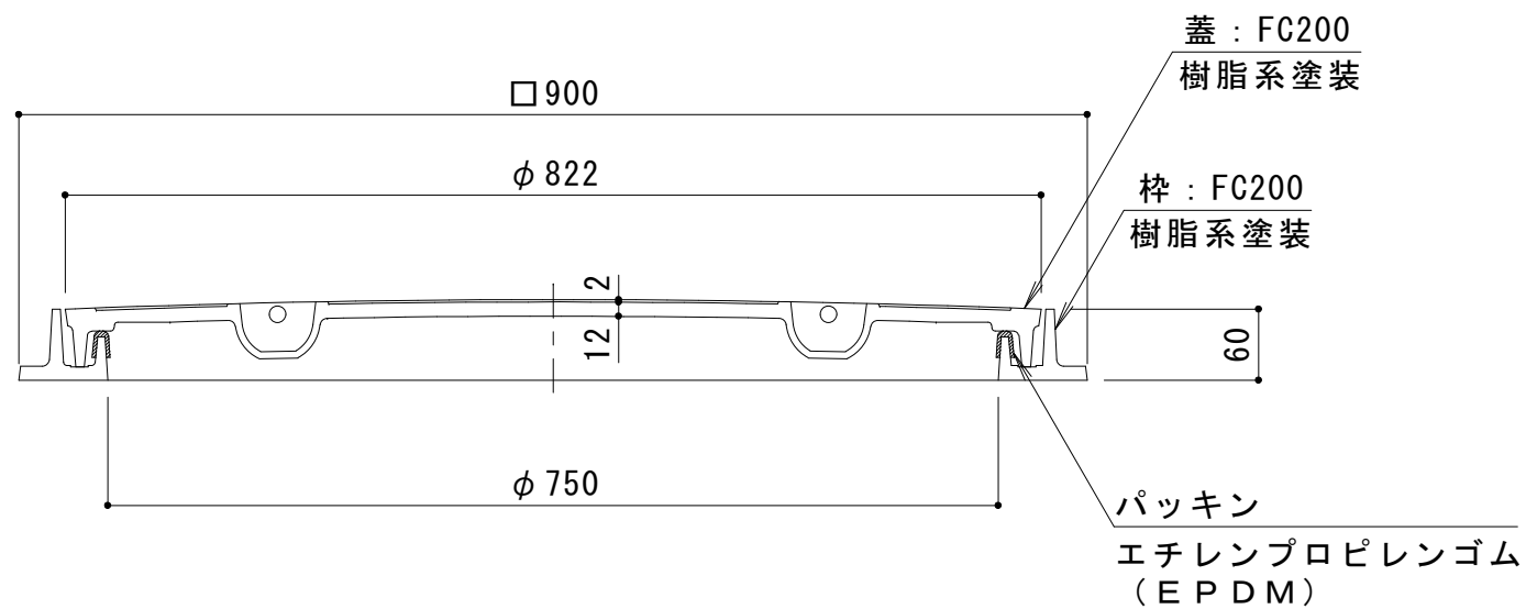
A-A断面図
