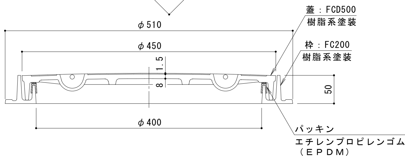
A-A断面図
