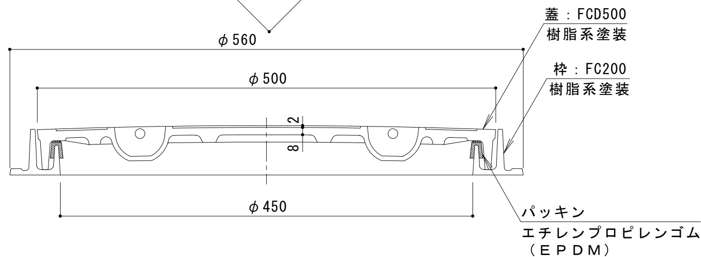
A-A断面図
