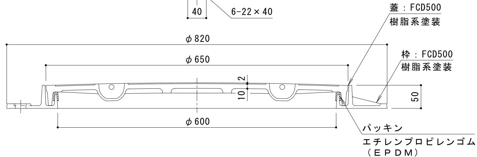
A-A断面図
