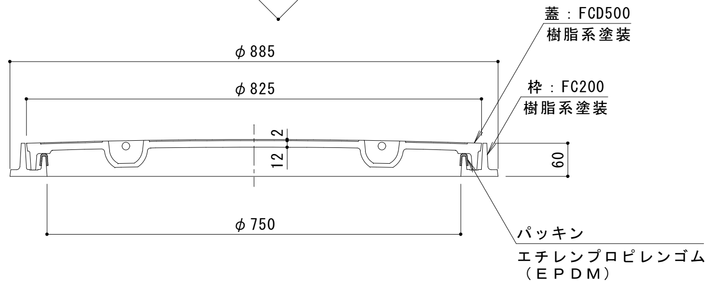
A-A断面図
