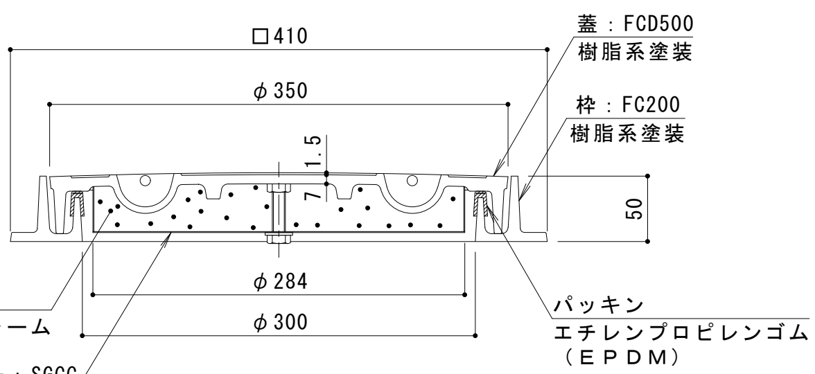
A-A断面図
