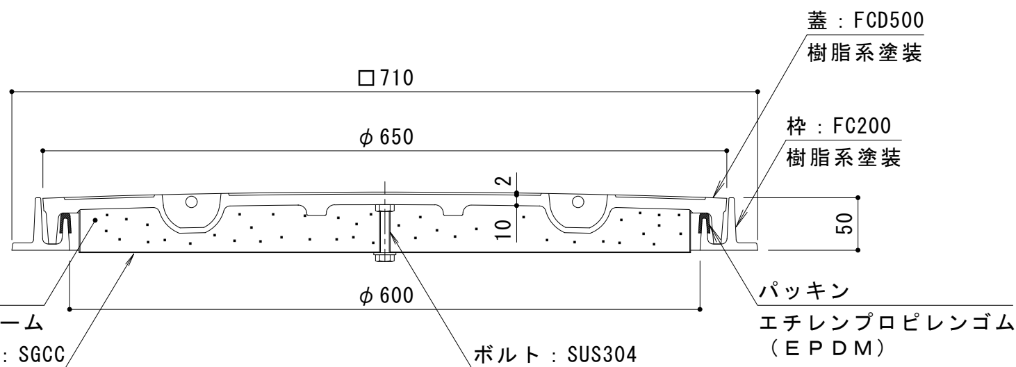
A-A 断面図
