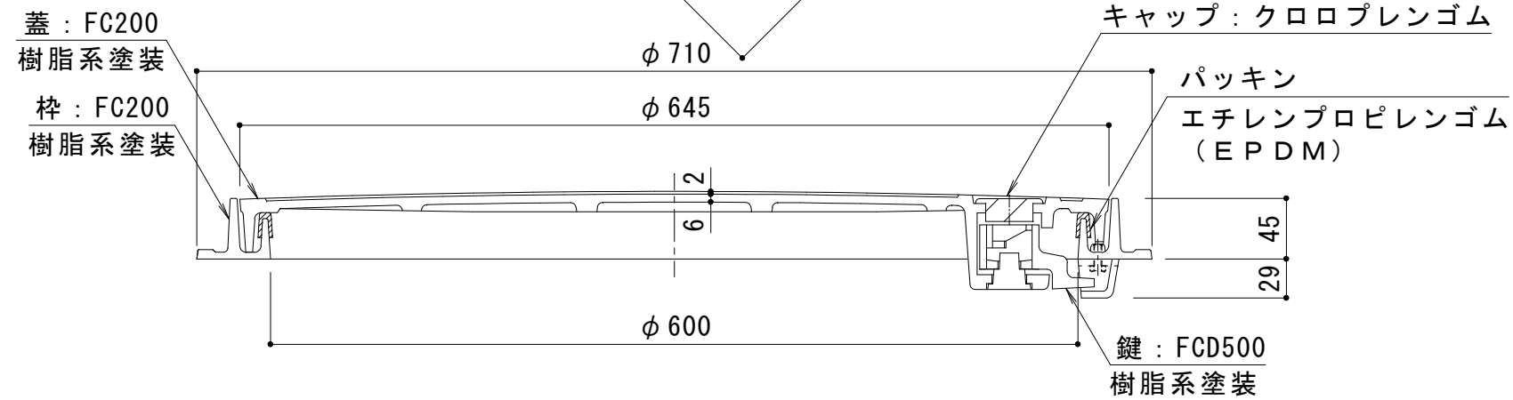
A-A断面図
