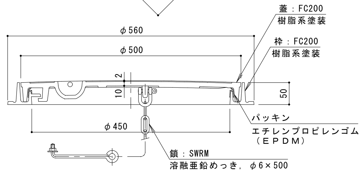
A-A断面図
