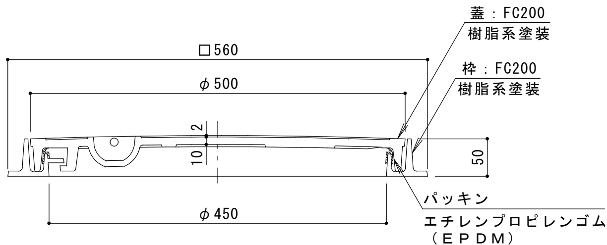
A-A断面図
