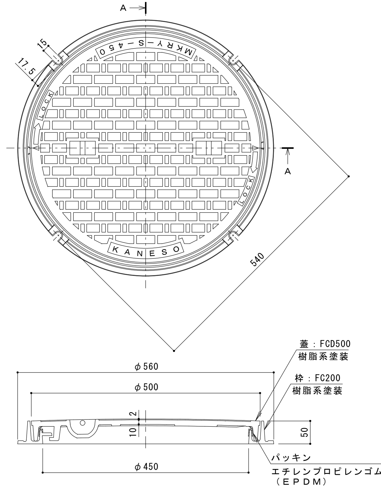
A-A断面図
