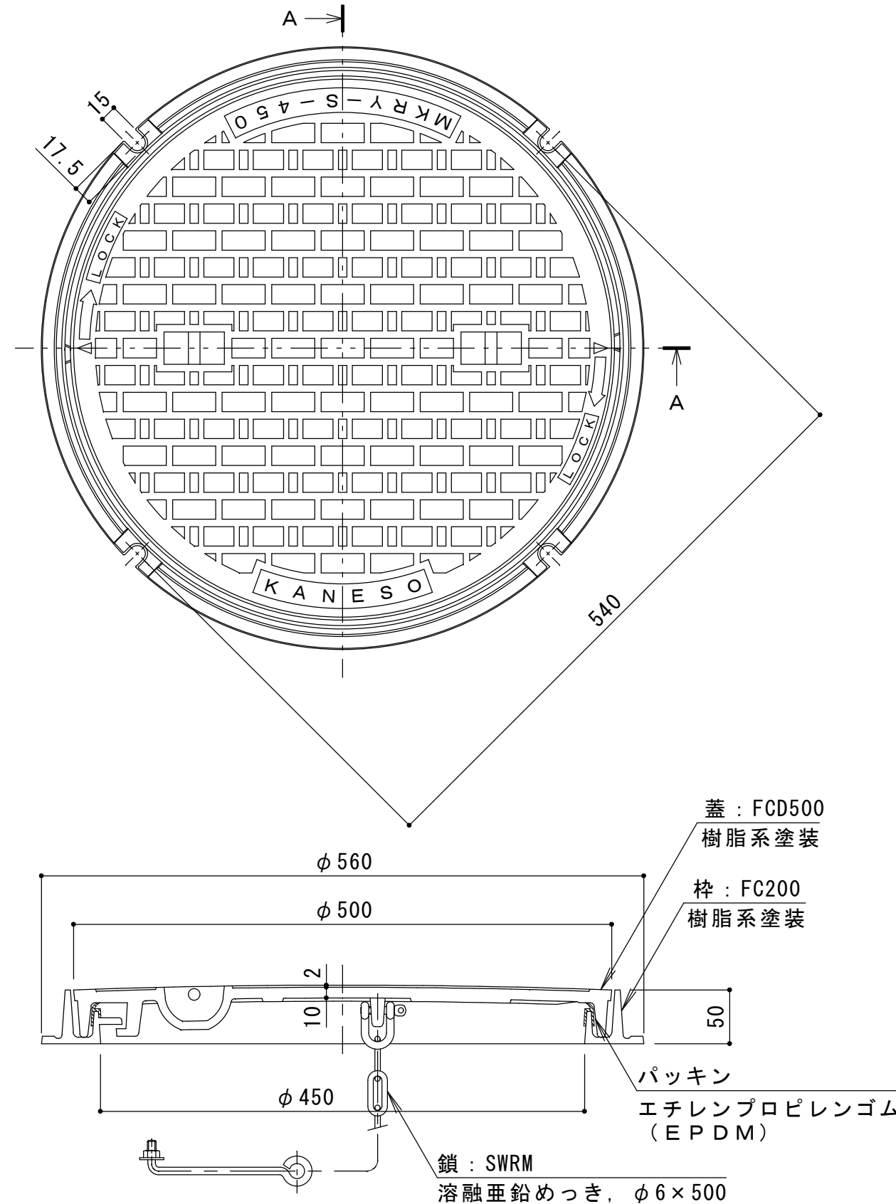
A-A断面図
