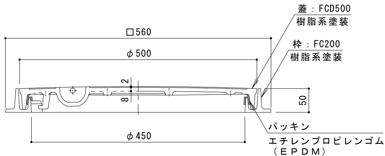
A-A断面図
