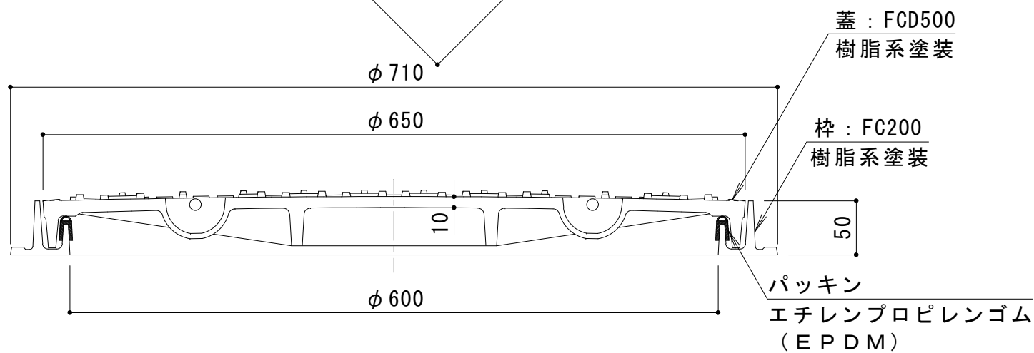
A-A 断面図
