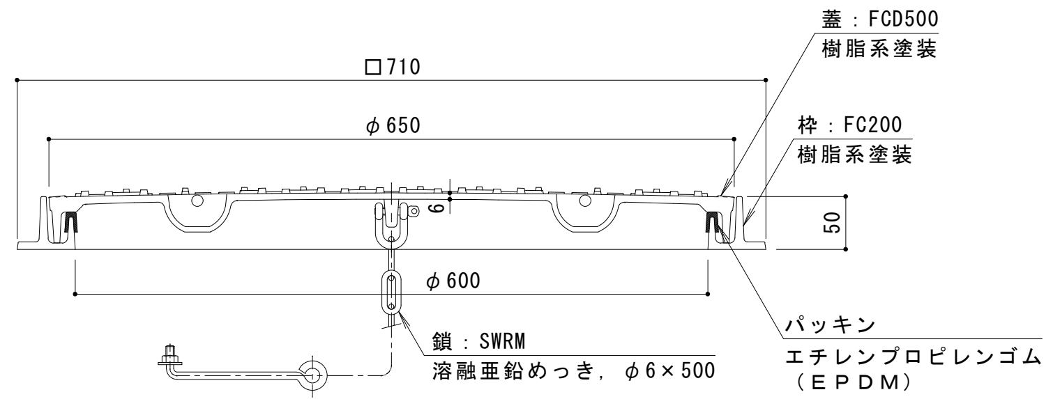
A-A断面図
