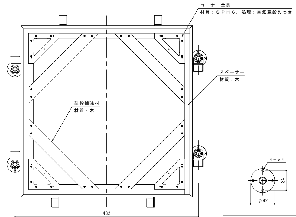
固定プレート平面図 S=1:2
