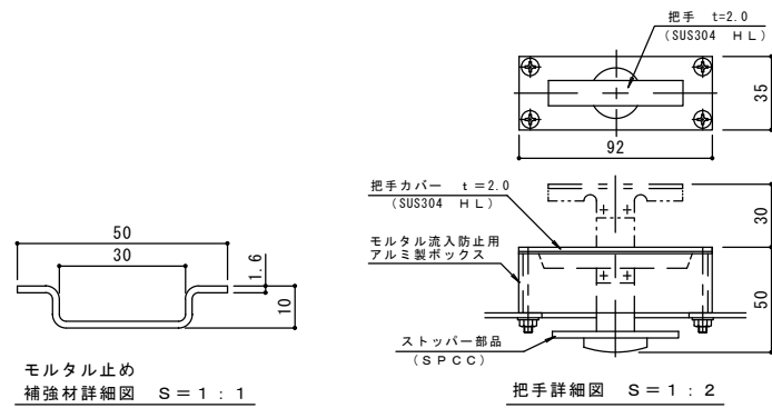
把手詳細図 S=1:2
