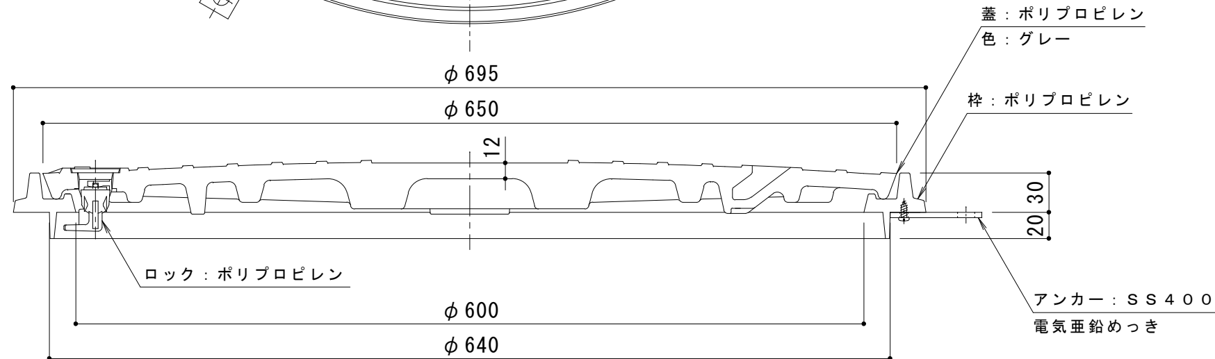
A-A断面図
